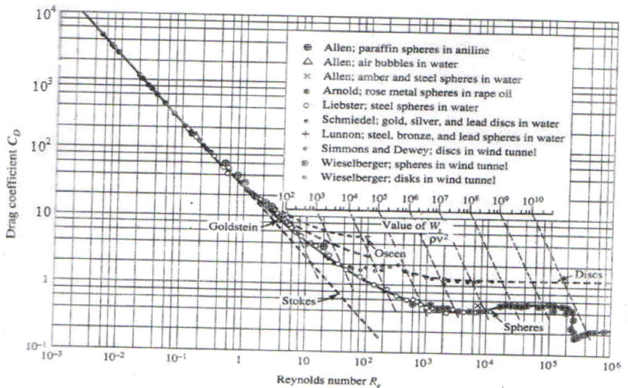
Fig. 2. Drag coefisien [10]
