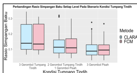
Gambar 12. Perbandingan nilai rasio simpangan baku antara metode CLARA dan FCM
