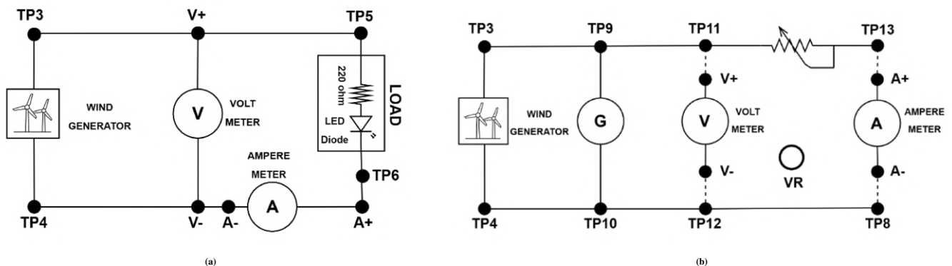
Gambar 6 (a) Diagram pengkabelan percobaan PLTB menggunakan beban tetap, (b) Diagram pengkabelan percobaan PLTB menggunakan beban variabel
