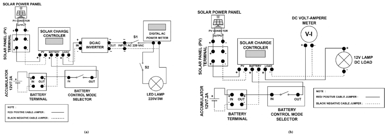
Gambar 4 (a) Diagram pengabelan untuk percobaan PLTS menggunakan beban AC, (b) Diagram pengabelan untuk percobaan PLTS menggunakan beban DC
