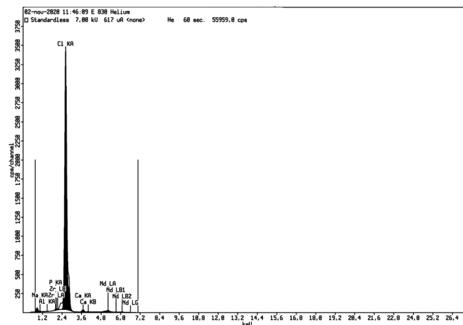
Gambar 5 Hasil uji XRF-Helium sampel garam tambak.
