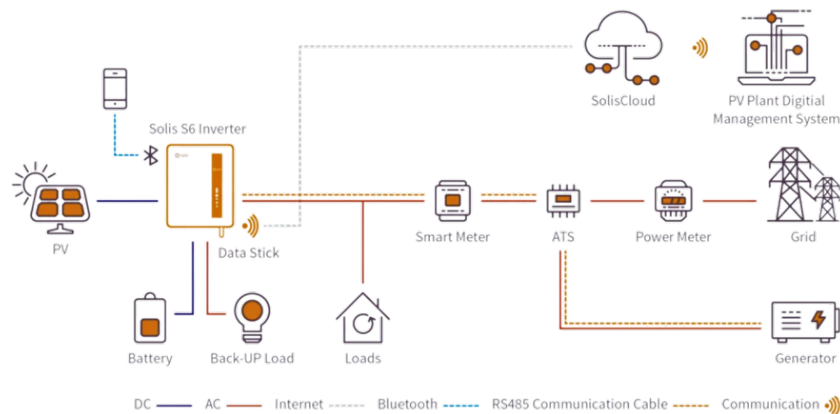
Gambar 1 Skema Sistem Solar Hybrid.
