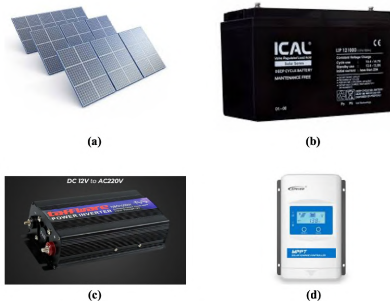
Gambar 2 Alat Pelatihan Instalasi PLTS: (a) Panel Surya; (b) Baterai; (c) Inverter 12 volt DC ke 220 Volt AC 50 Hz; (d) Pengendali Pengisian berbasis MPPT
